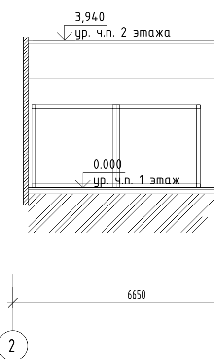
Фрагмент Коридор с местом установки холодильного оборудования пом.14.7.1 разрез 1-1
