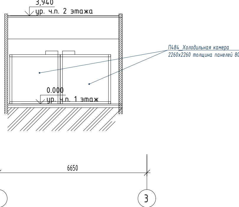
Фрагмент Коридор с местом установкой холодильного оборудования пом.14.71 разрез 1-1
