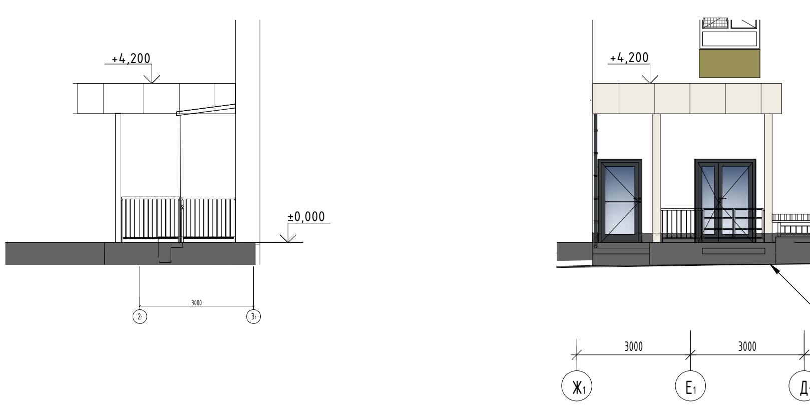
Фрагмент Габаритный размеры и высоты козырька
